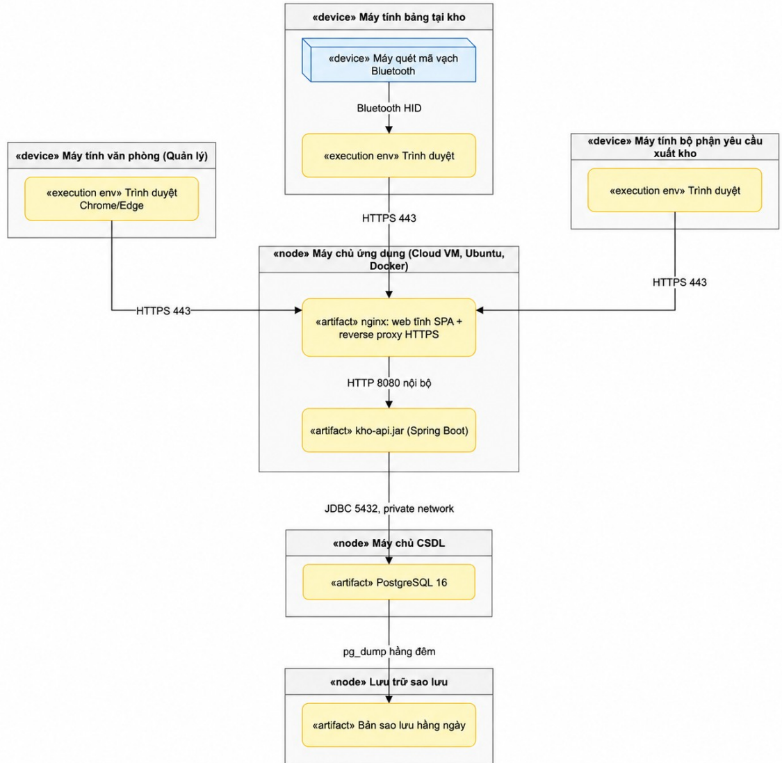
Hình 3. Thiết kế triển khai đề xuất
